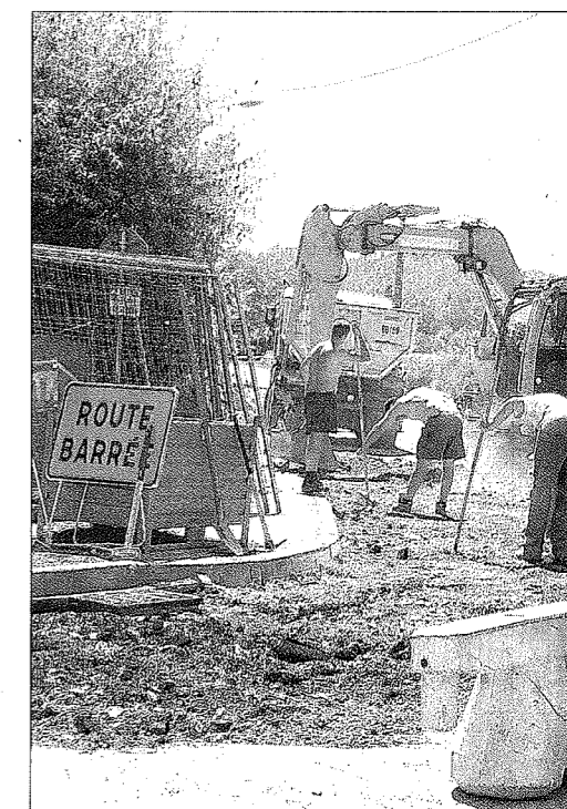
Sur le chantier des réseaux humides, chemin des Casernes.
